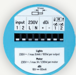
dDi Base (für DALI)
